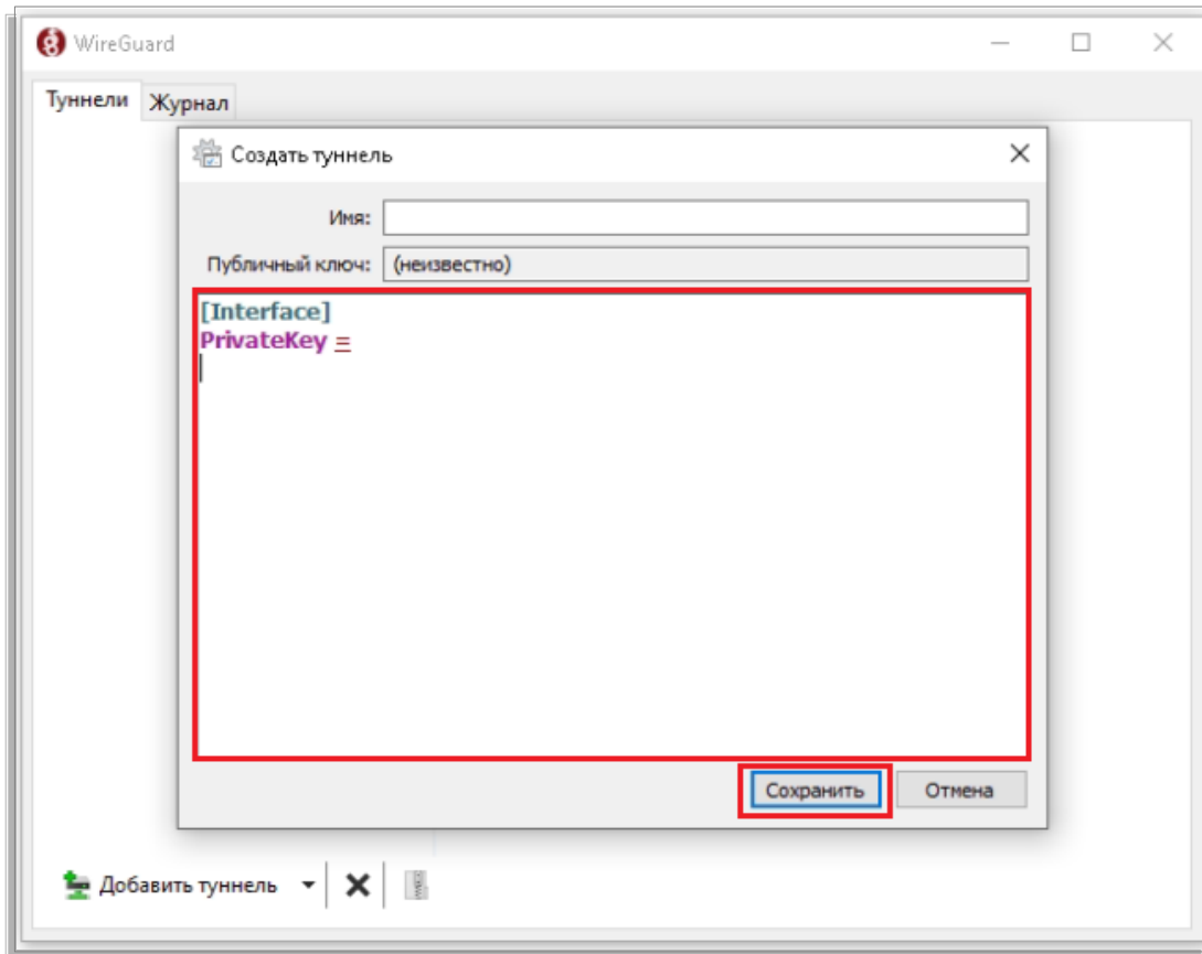
Рисунок 18. Заполнение туннеля в WireGuard
